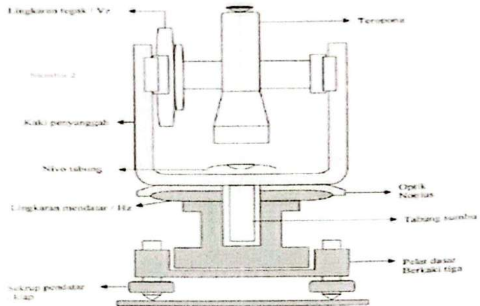
Gambar 2.3 Teodolit
